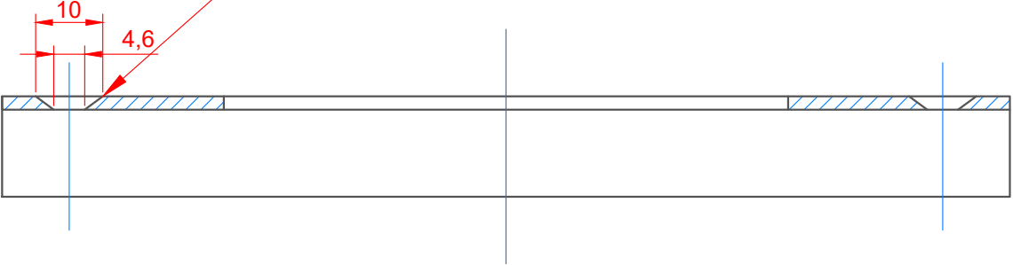
Вид В-В
