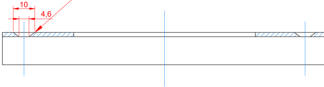
Вид В-В
